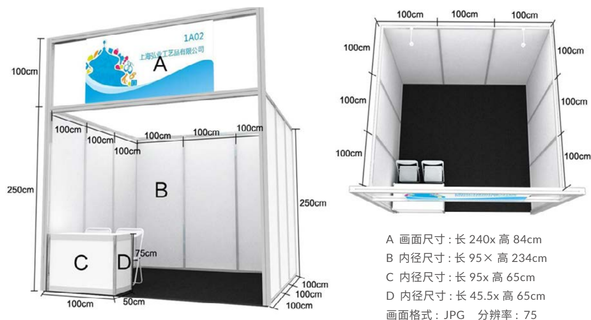
豪标尺寸图
